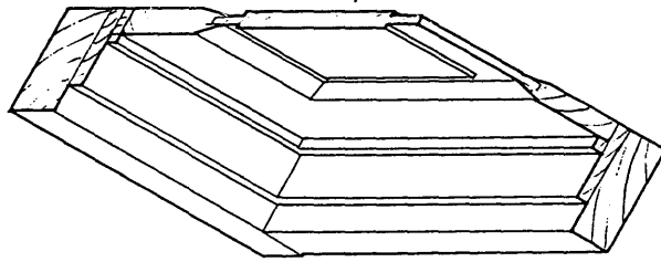
B. DOOR LAMB DETAIL
